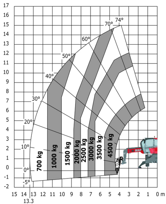
Machine sur stabilisateurs abaissés avec treuil 5000 kg
