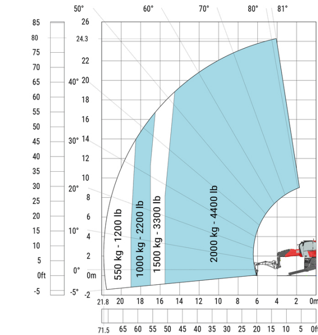
Machine sur stabilisateurs abaissés avec potence 2000 kg (Imperial)
