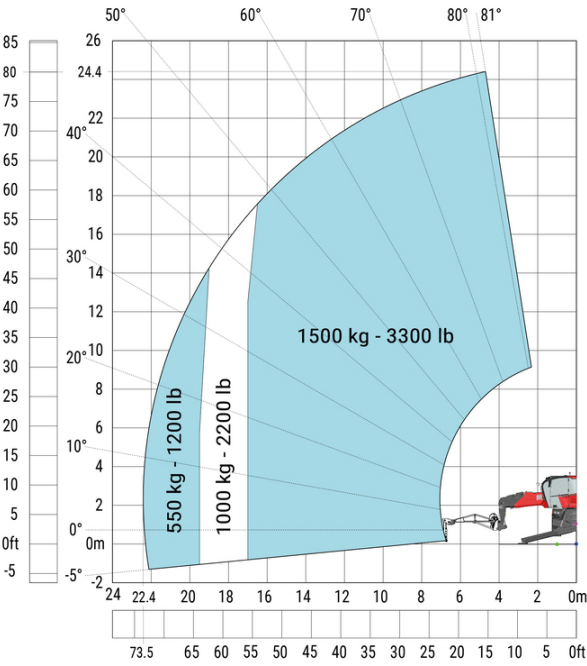
Machine sur stabilisateurs abaissés avec potence 1500 kg Machine sur stabilisateurs abaissés avec potence 1500 kg Impérial
