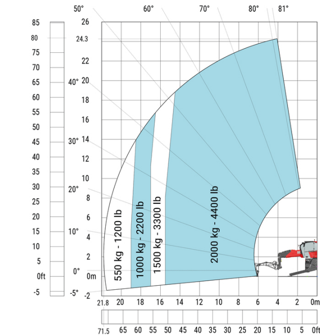
Machine sur stabilisateurs abaissés avec potence 2000 kg (Métrique)
